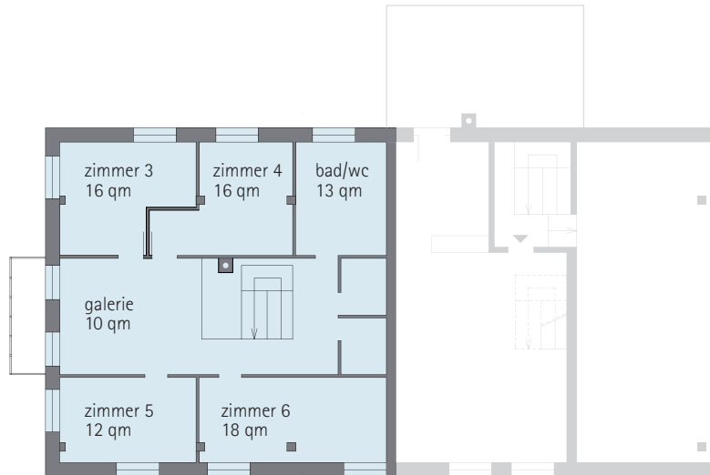
obergeschoss
